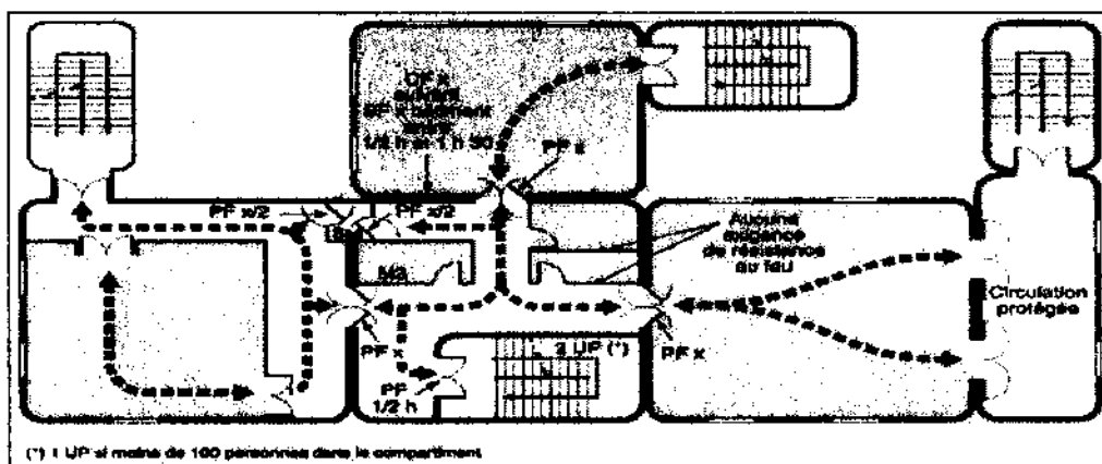
Exemple de quatre compartiments en plan
